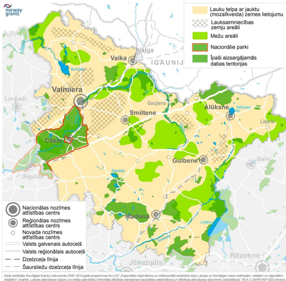
4.2.3. attēls Lauksaimniecības telpas, mežu telpas, lauku telpas ar jauktu (mozaikveida) lietojumu 2030
